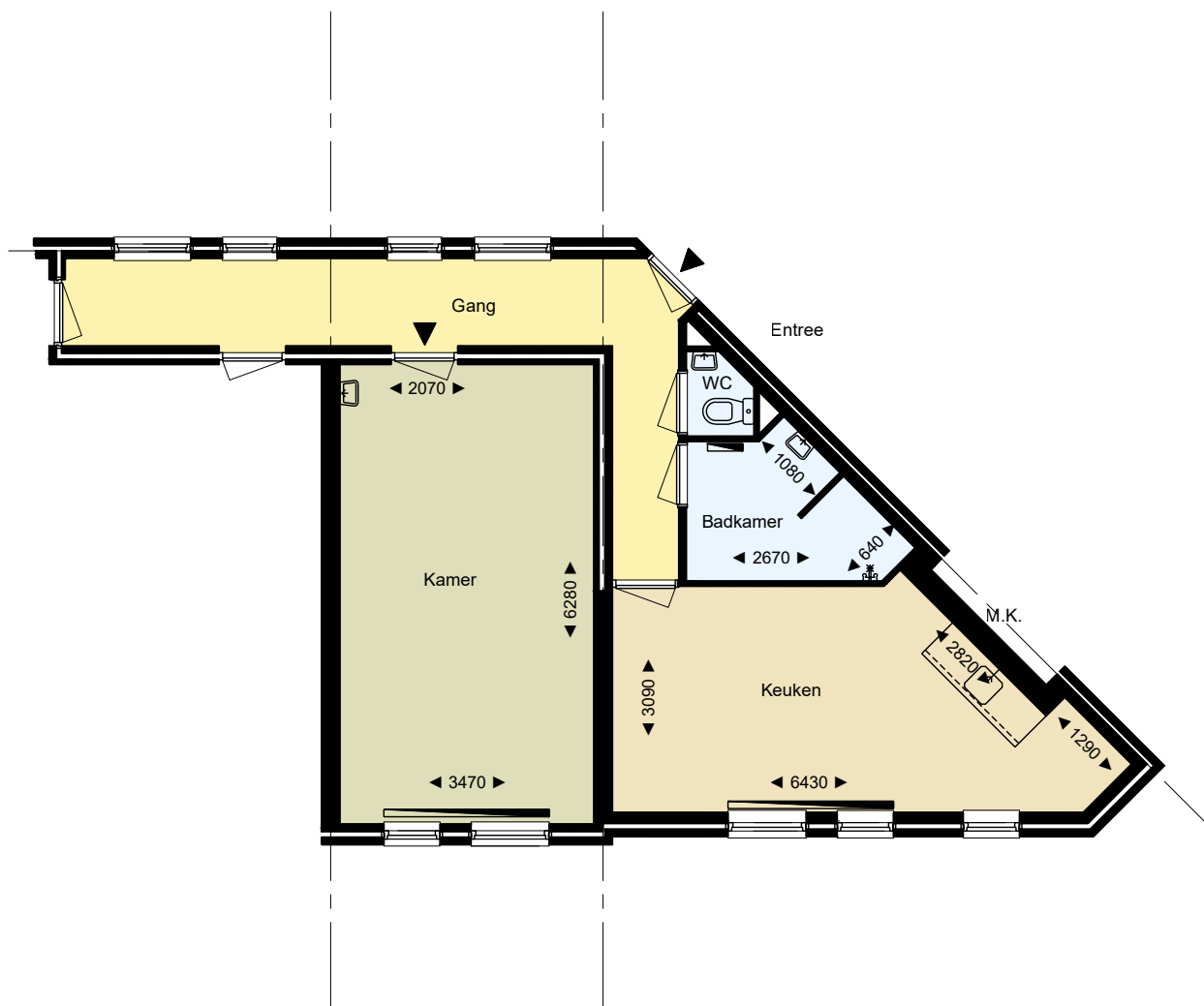
Begane grond schaal 1:100
